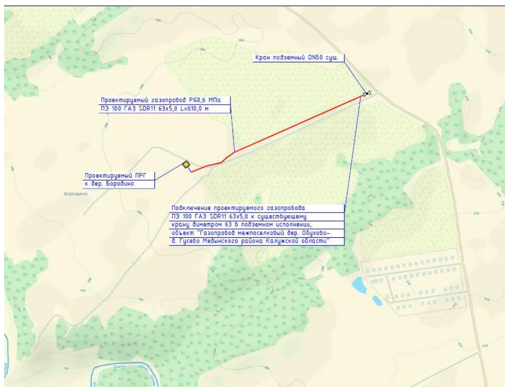
Рисунок 3.1 – Обзорная схема участка строительства
